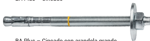
BA Plus – Cincado con arandela grande
