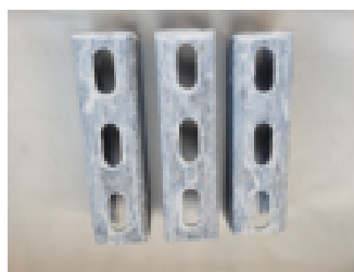
Probetas a 1000 horas en NSS
